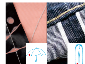
链式线迹
